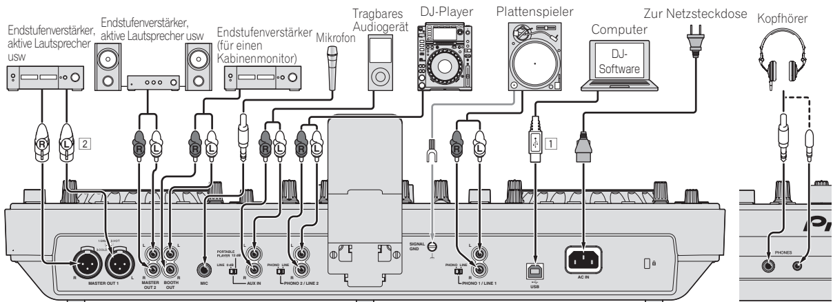
Rückseite
