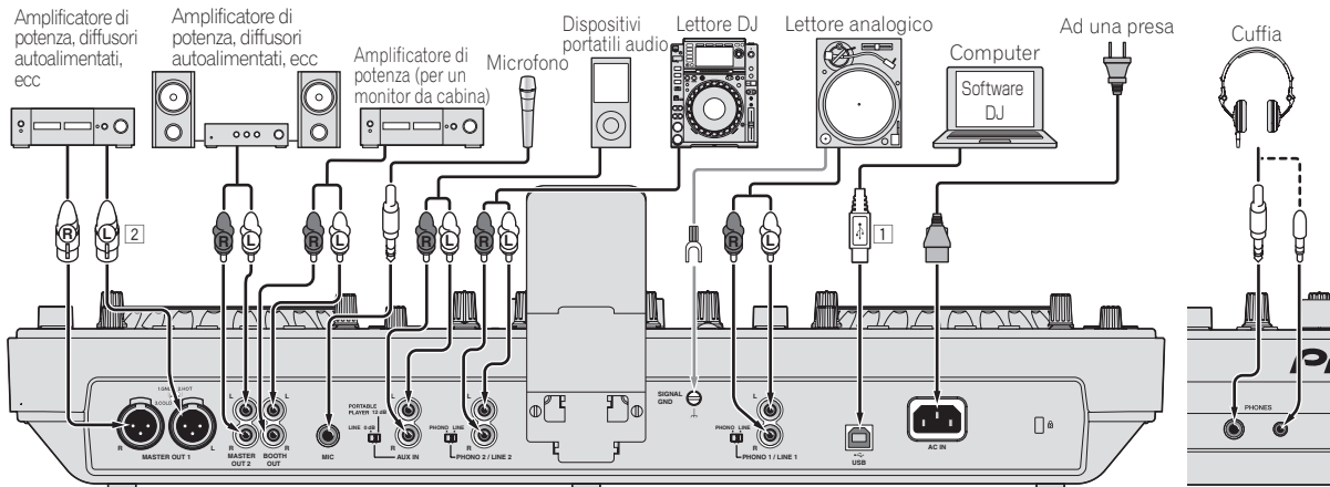
Pannello posteriore
