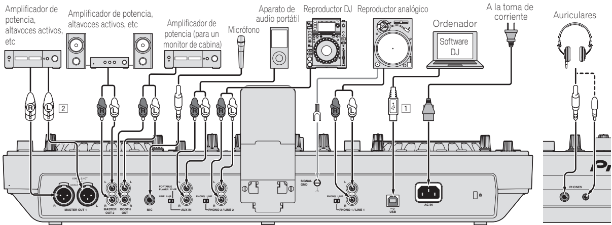
Panel posterior
