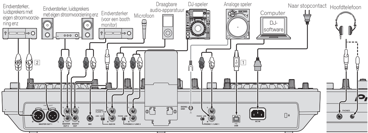
Achterpaneel
