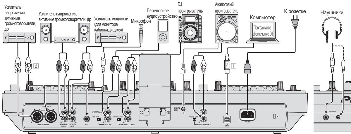
Задняя панель
