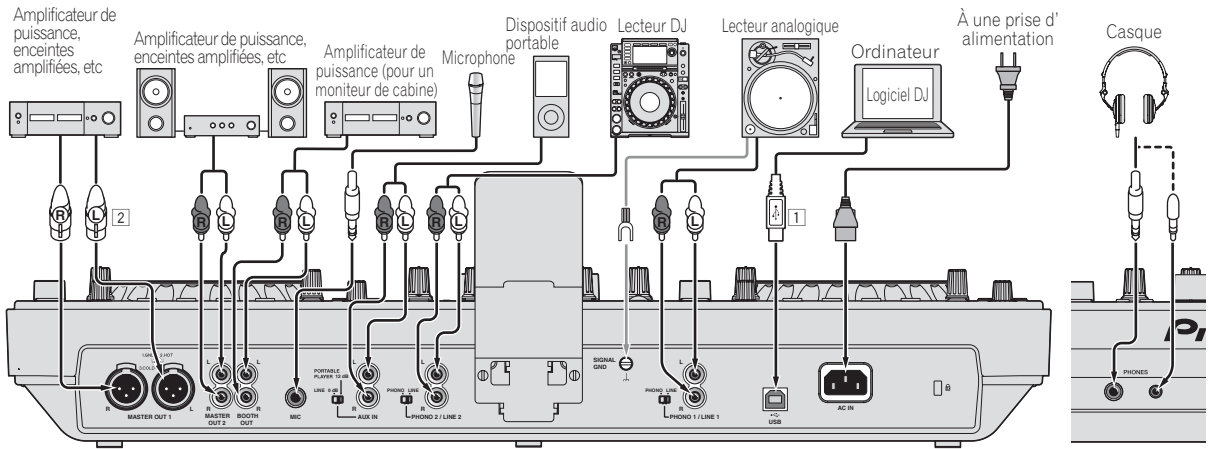
Panneau arrière
