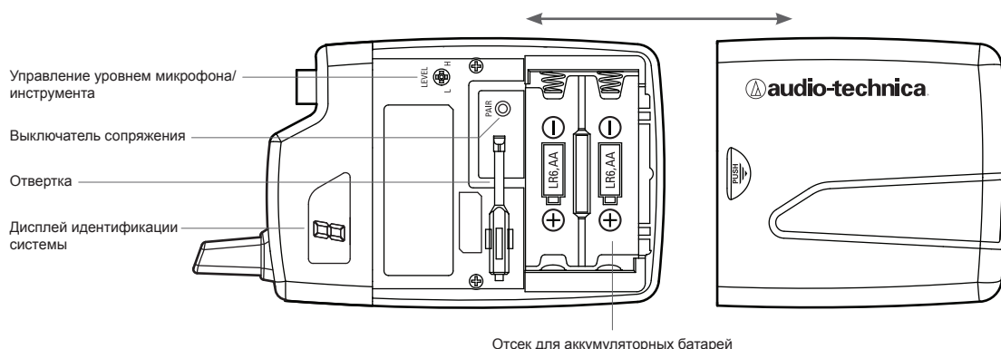
Рисунок D — Передатчик ATW-T1001EX UniPak®
