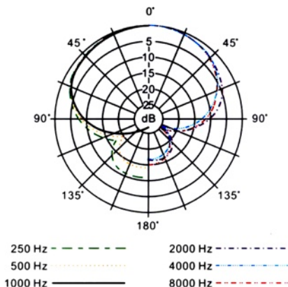
Диаграмма направленности
