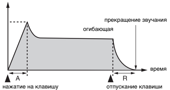
A — время нарастания R — время затухания
