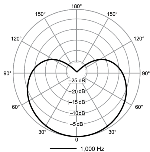
Диаграмма направленности
