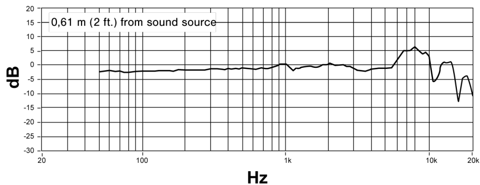
Амплитудно-частотная характеристика
