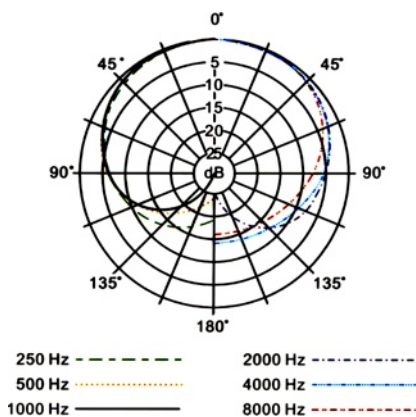
Диаграмма направленности
