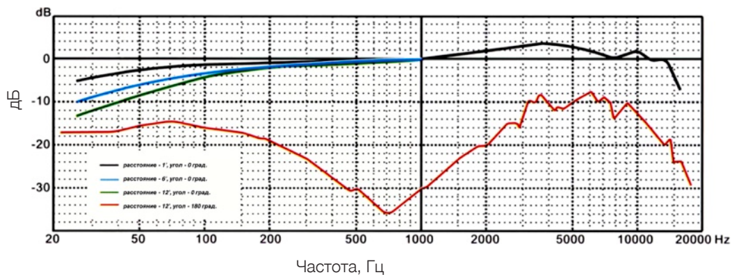
Частотный диапазон
